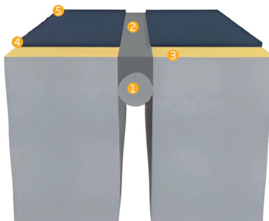
ОБРОБКА З'ЄДНАНЬ ГЕРМЕТИКОМ
